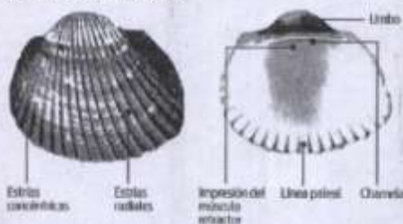
Diagrama de la cara interna y externa de las valvas de un molusco bivalve.
