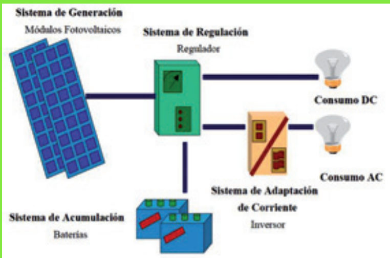
Método de funcionamiento de la energía mecánica fotovoltaica
