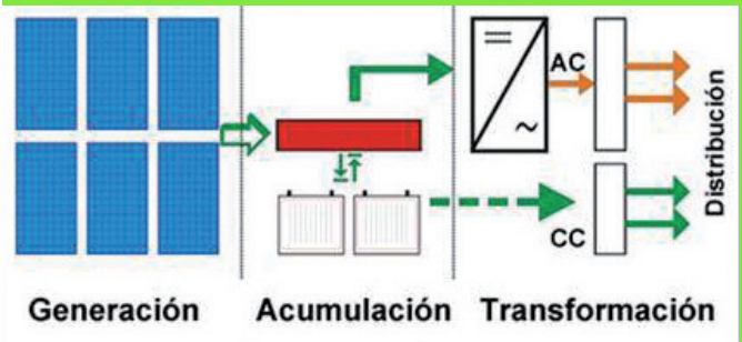
Método de funcionamiento de la energía mecánica fotovoltaica
