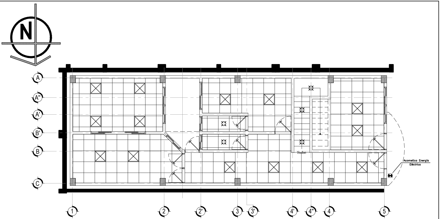
Cielo Reflejado - Primer Nivel ESC. 1:100
