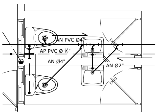
Detalle Baño Primer Nivel
