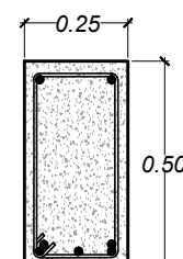
VIGA V-1
