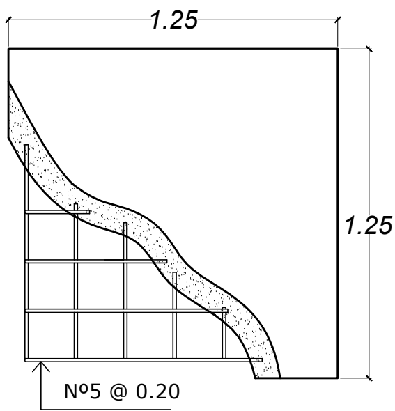
ZAPATA Z-1
