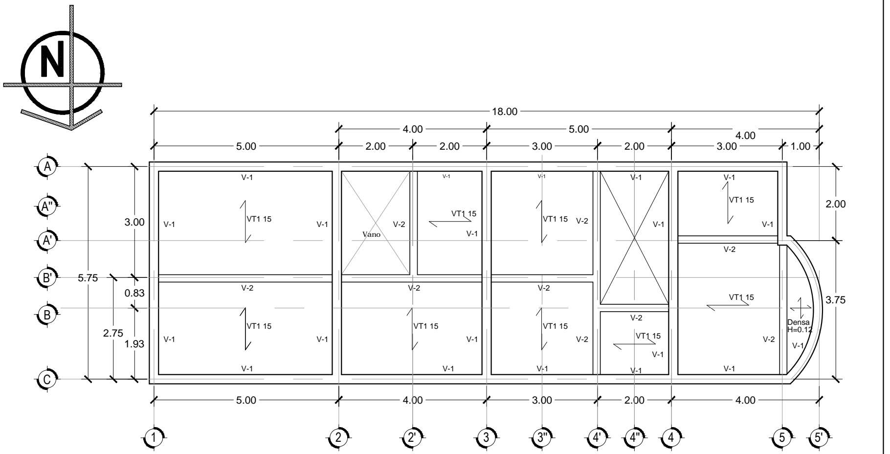
Planta Estructural de Entrepiso ESC. 1:100
