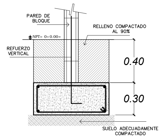
DETALLE DE SOLERA CON PARED
