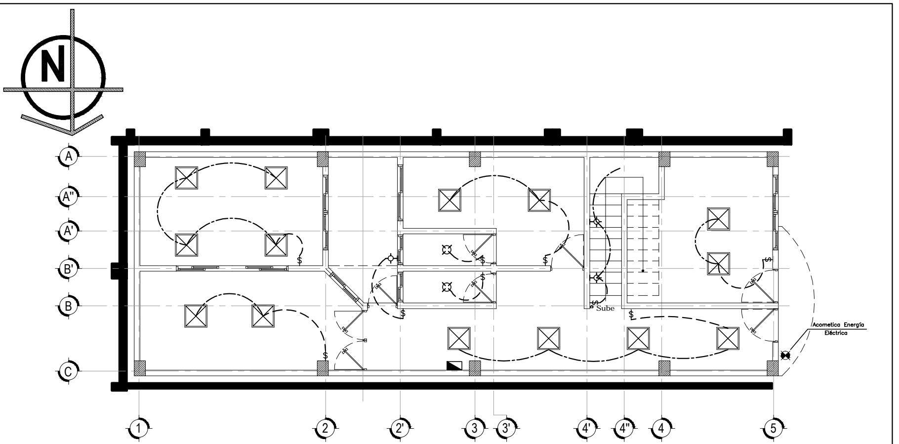
Luminarias - Primer Nivel ESC. 1:100
