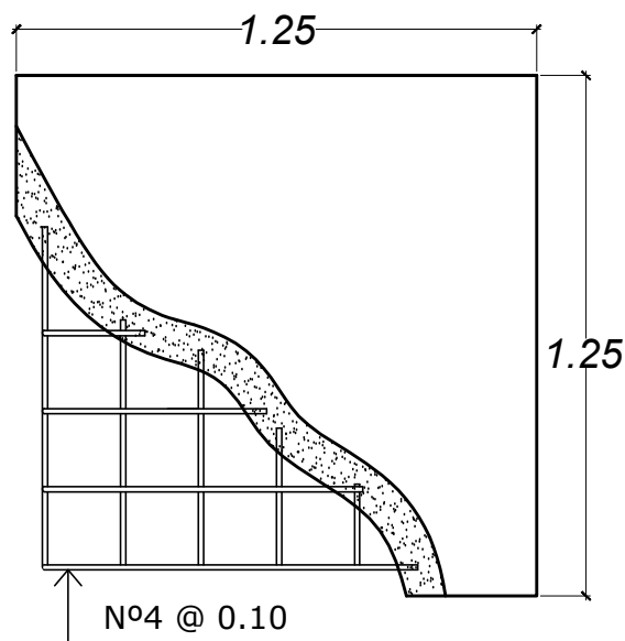
ZAPATA Z-1
