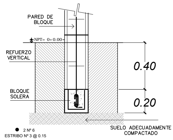
DETALLE DE SOLERA SF-2 CON PARED
