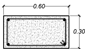
SOLERA DE FUNDACION S-1
