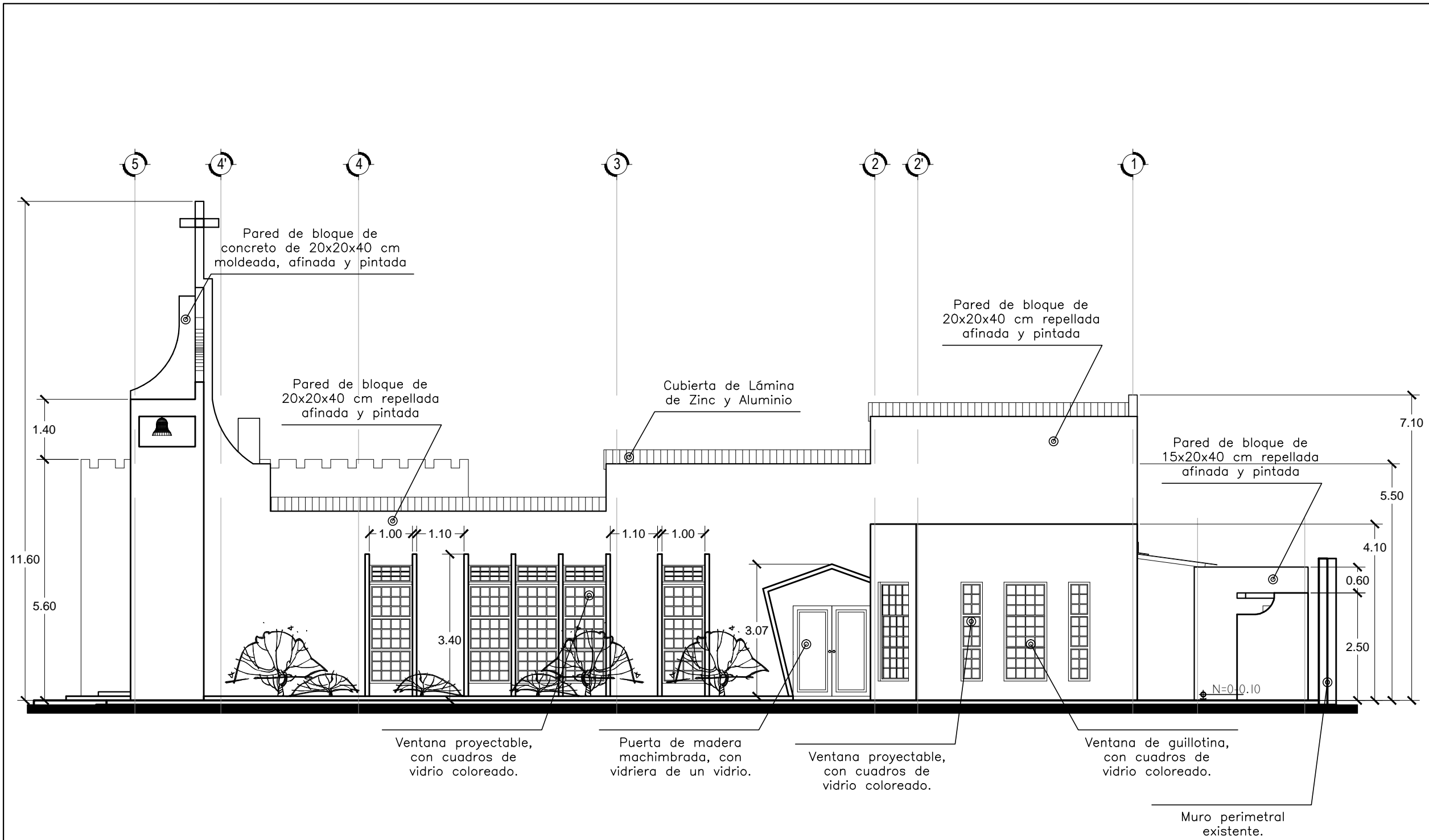
Fachada Poniente ESC. 1:100
