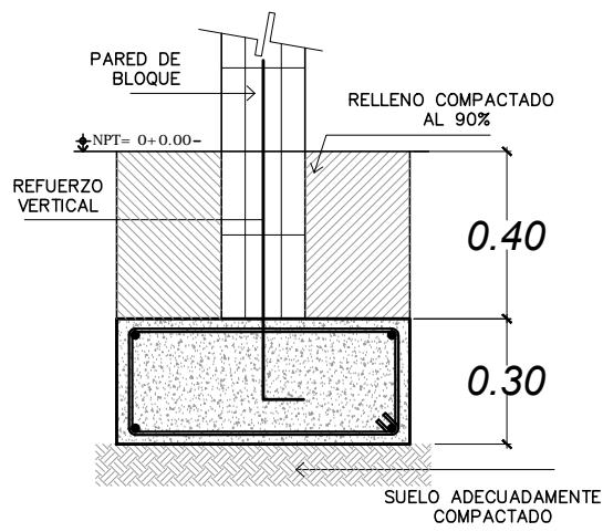
DETALLE DE SOLERA SF-1 CON PARED
