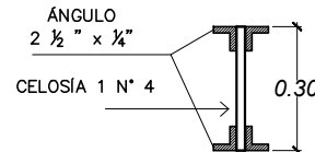
VIGA VM-1
