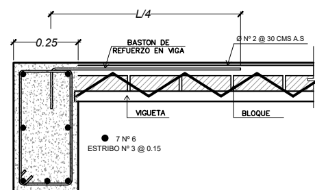
DETALLE DE APOYO DE VIGUETA EN VIGAS
