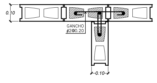
JUNTA T E
