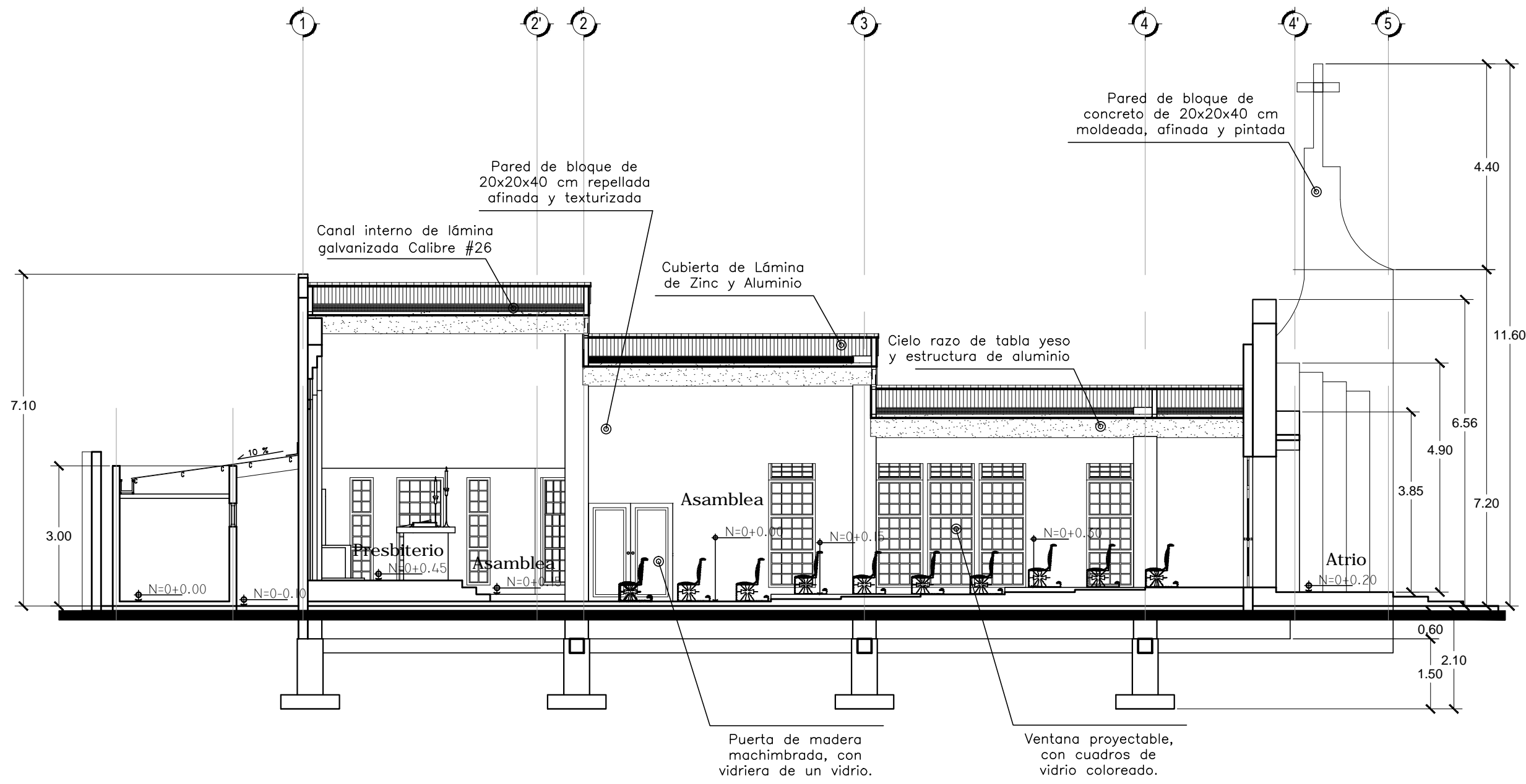
Corte Longitudinal A-A ESC. 1:100
