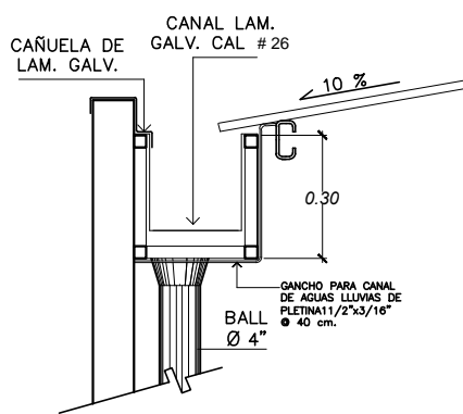
DETALLE CANAL INTERNO
