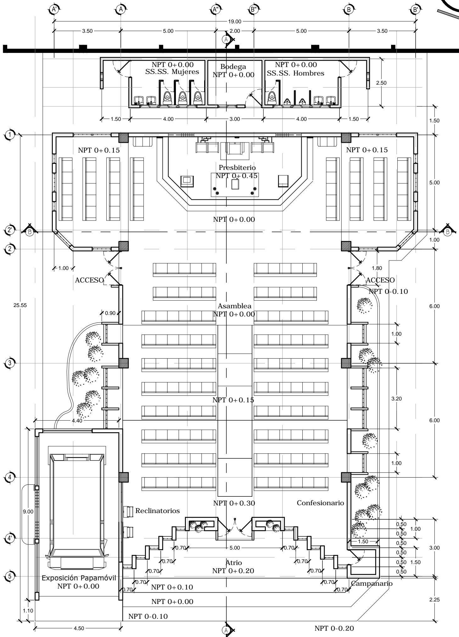
Planta Arquitectónica Capilla ESC. 1:125
