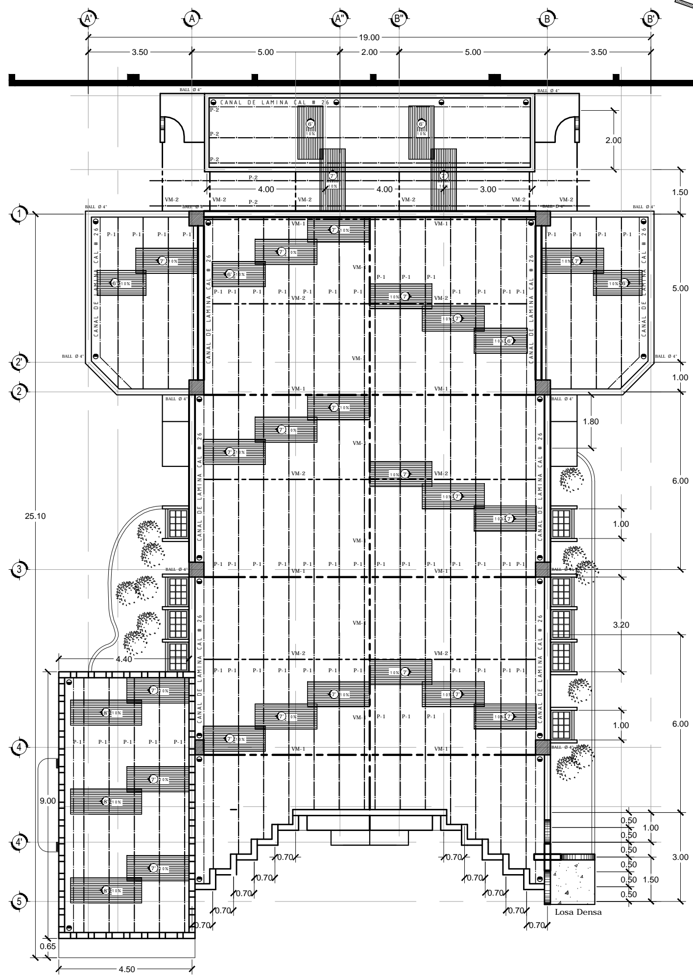
Planta Estructural de Techos - Capilla ESC. 1:125
