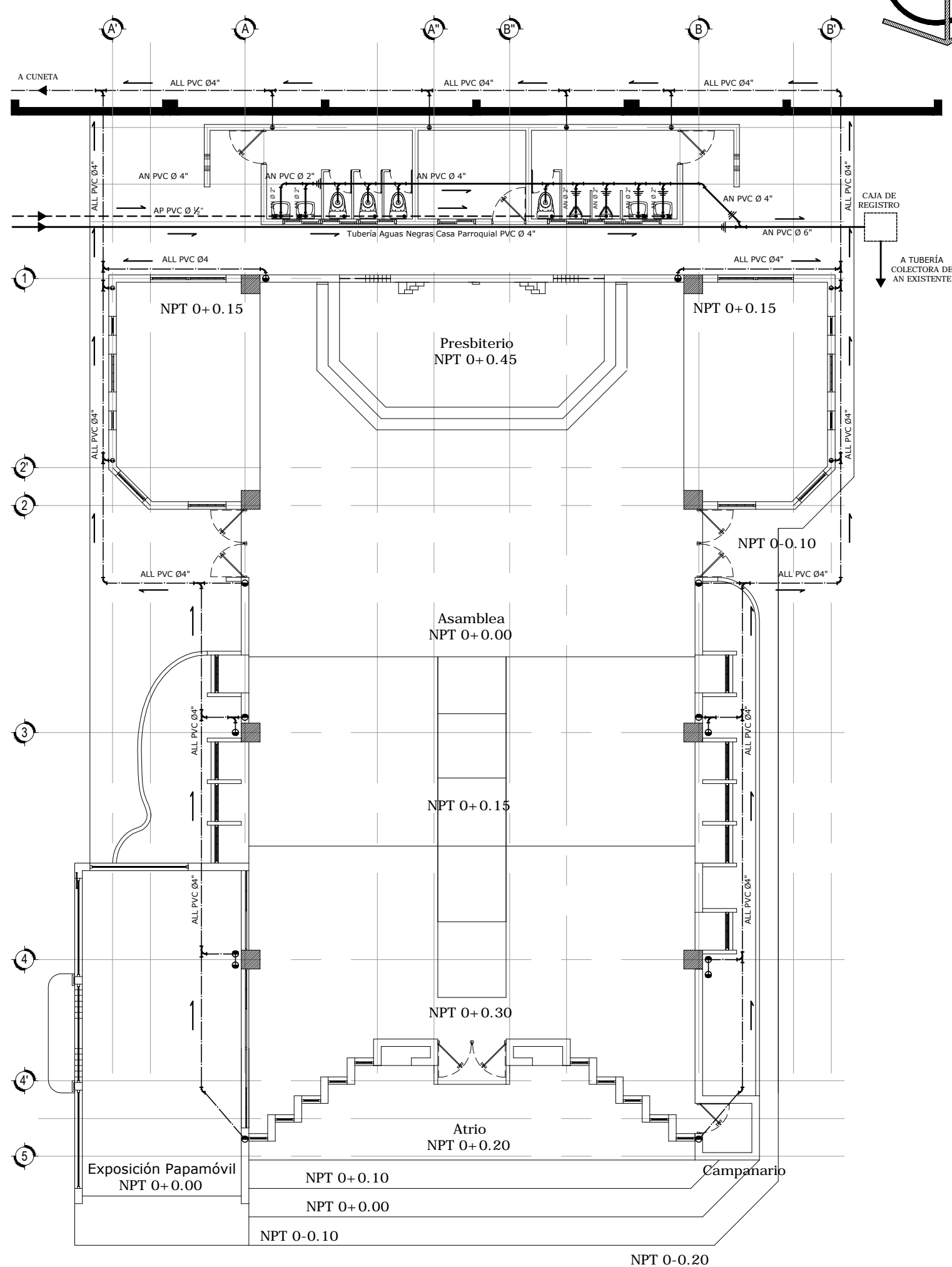
Planta de Instalaciones Hidráulicas ESC. 1:125
