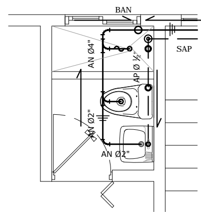
Detalle Baño Dormitorio Principal
