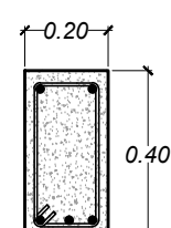
VIGA V-2
