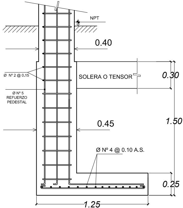
DESPLANTE DE FUNDACIONES
