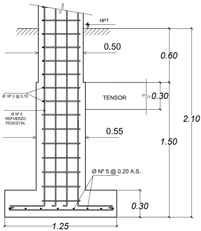
DESPLANTE DE FUNDACIONES
