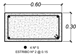
SOLERA DE FUNDACION S-1
