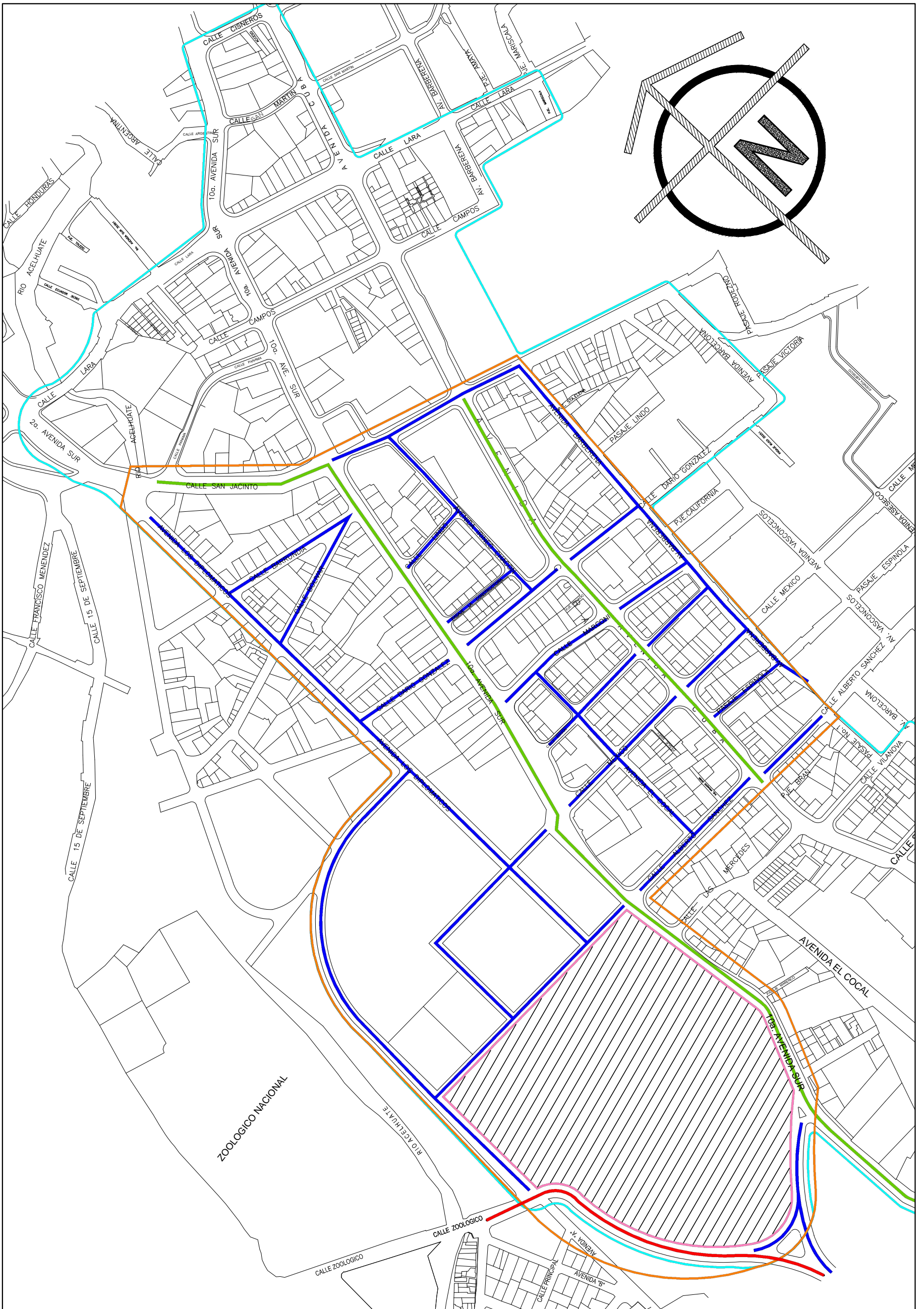
Plano de Jerarquización Vial - Esc.: 1/4000
