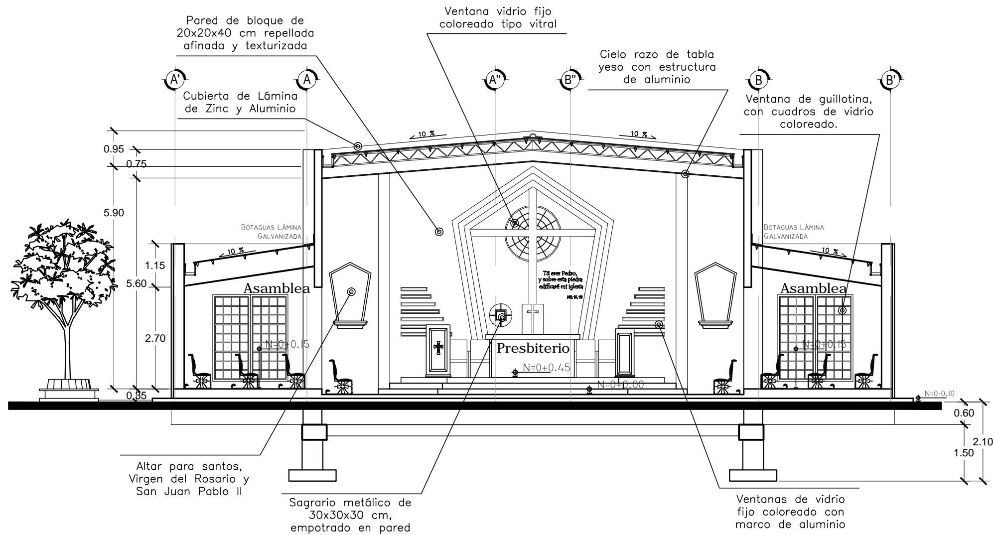
Corte Transversal B-B ESC. 1:100
