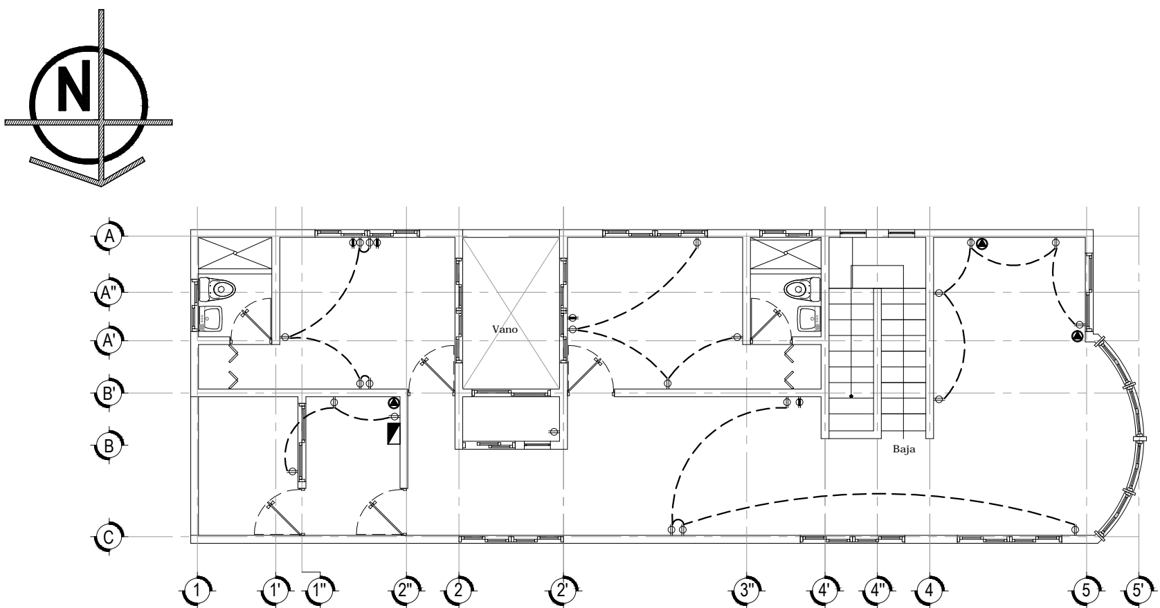
Tomas Eléctricos - Primer Nivel ESC. 1:100
