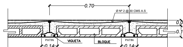
SISTEMA LOSA COPRESA TRADICIONAL DETALLE DE LOSA TIPO VT1-15
