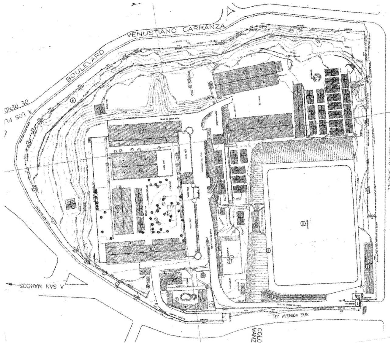
PLN340101: Plano Topográfico – Esc 1:2000 Fuente: Biblioteca Especializada de Historia Militar – Centro de Historia Militar
