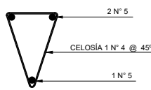
POLÍN P-1
