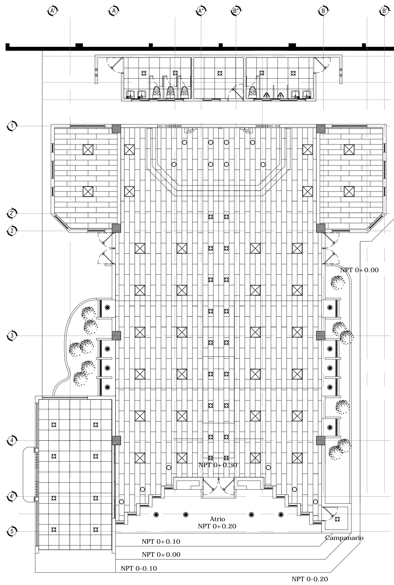
Cielo Reflejado ESC. 1:125
