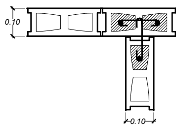
JUNTA DESFASADA
