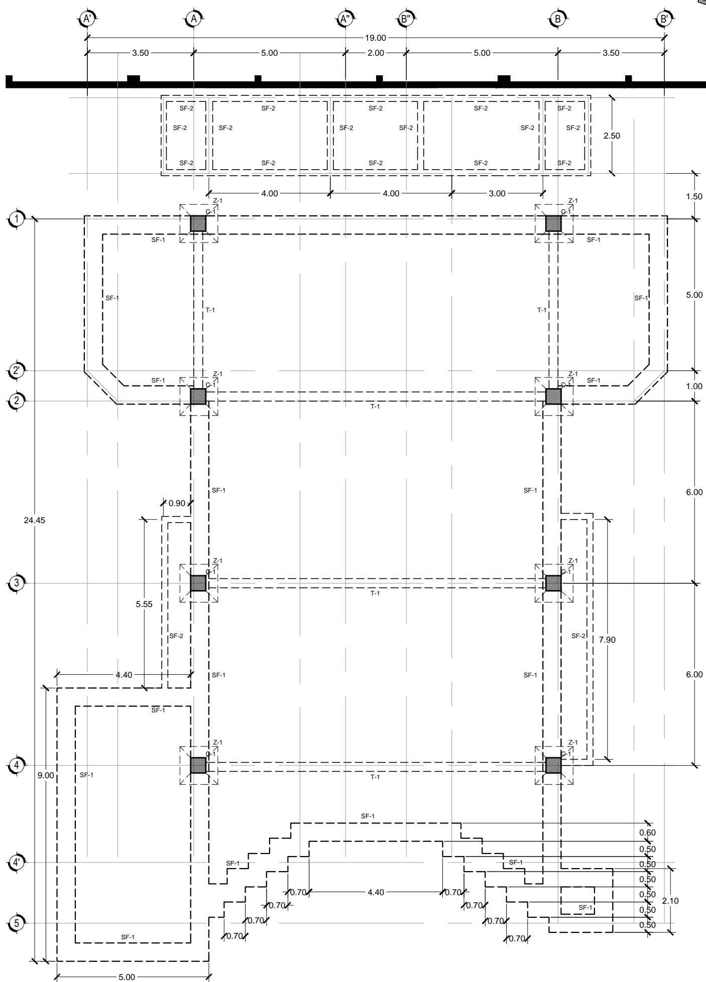
Planta de Fundaciones - Capilla ESC. 1:125
