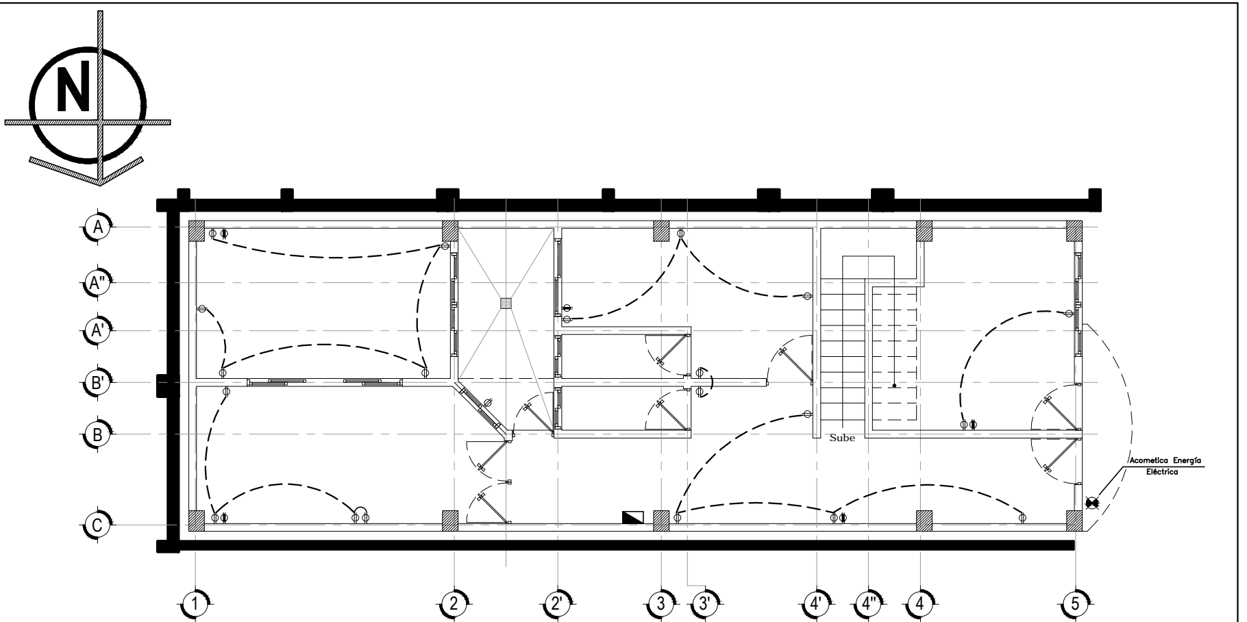
Tomas Eléctricos - Primer Nivel ESC. 1:100
