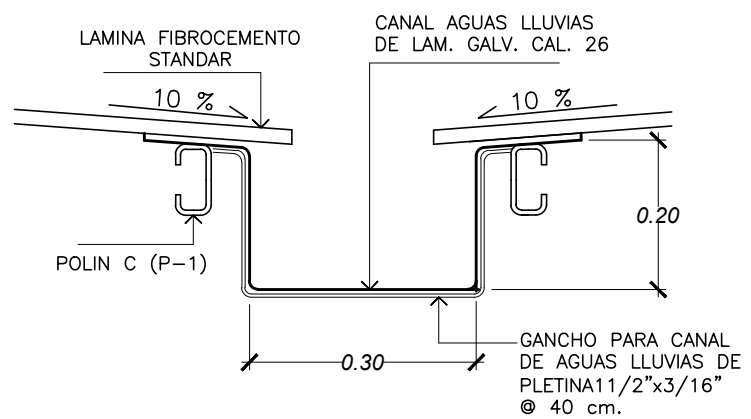
DETALLE DE CANAL
