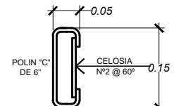
VIGA VM-2
