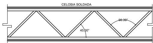
DETALLE VIGA VM-1 DE ALMA ABIERTA
