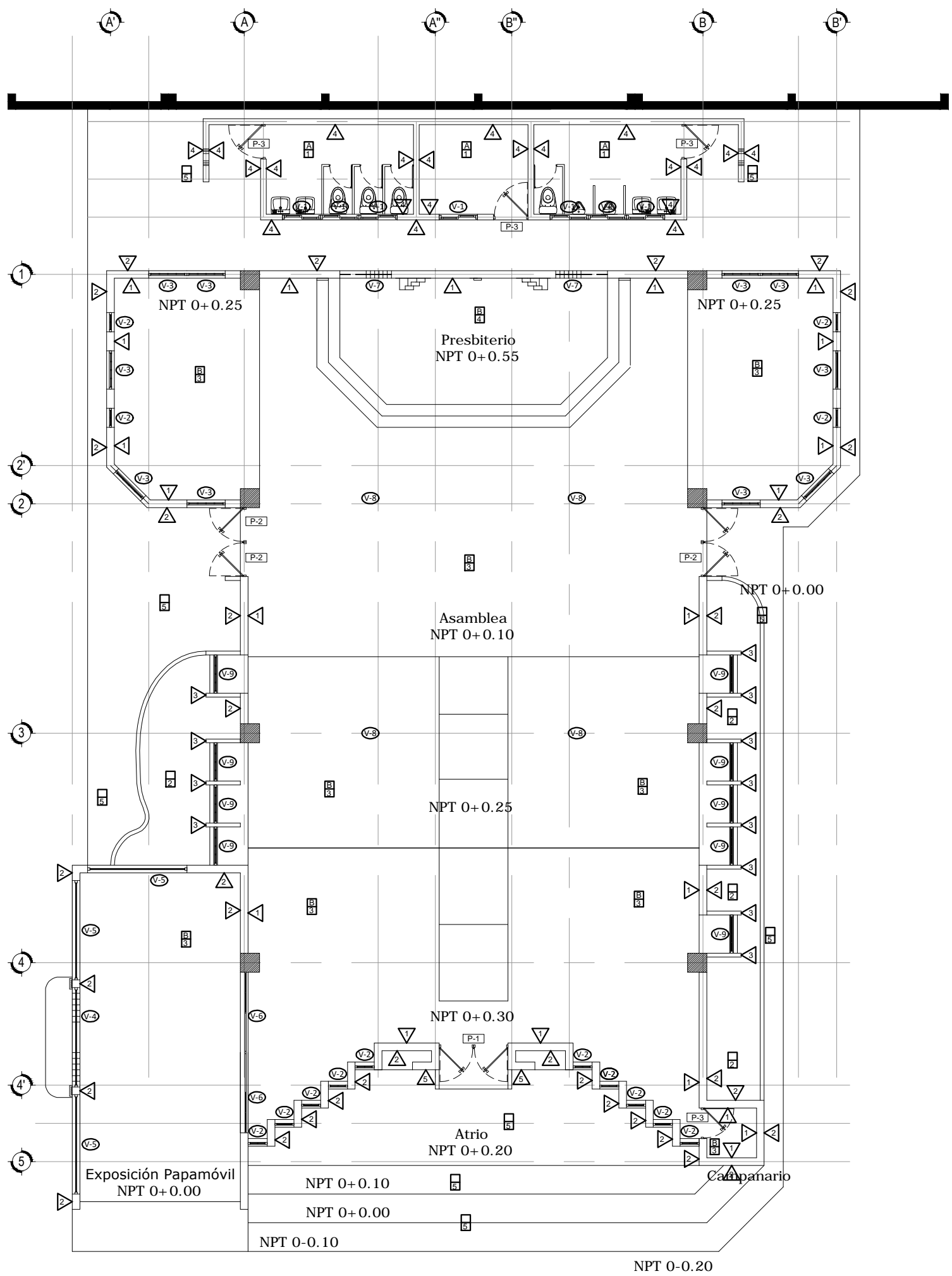
Planta de Acabados
