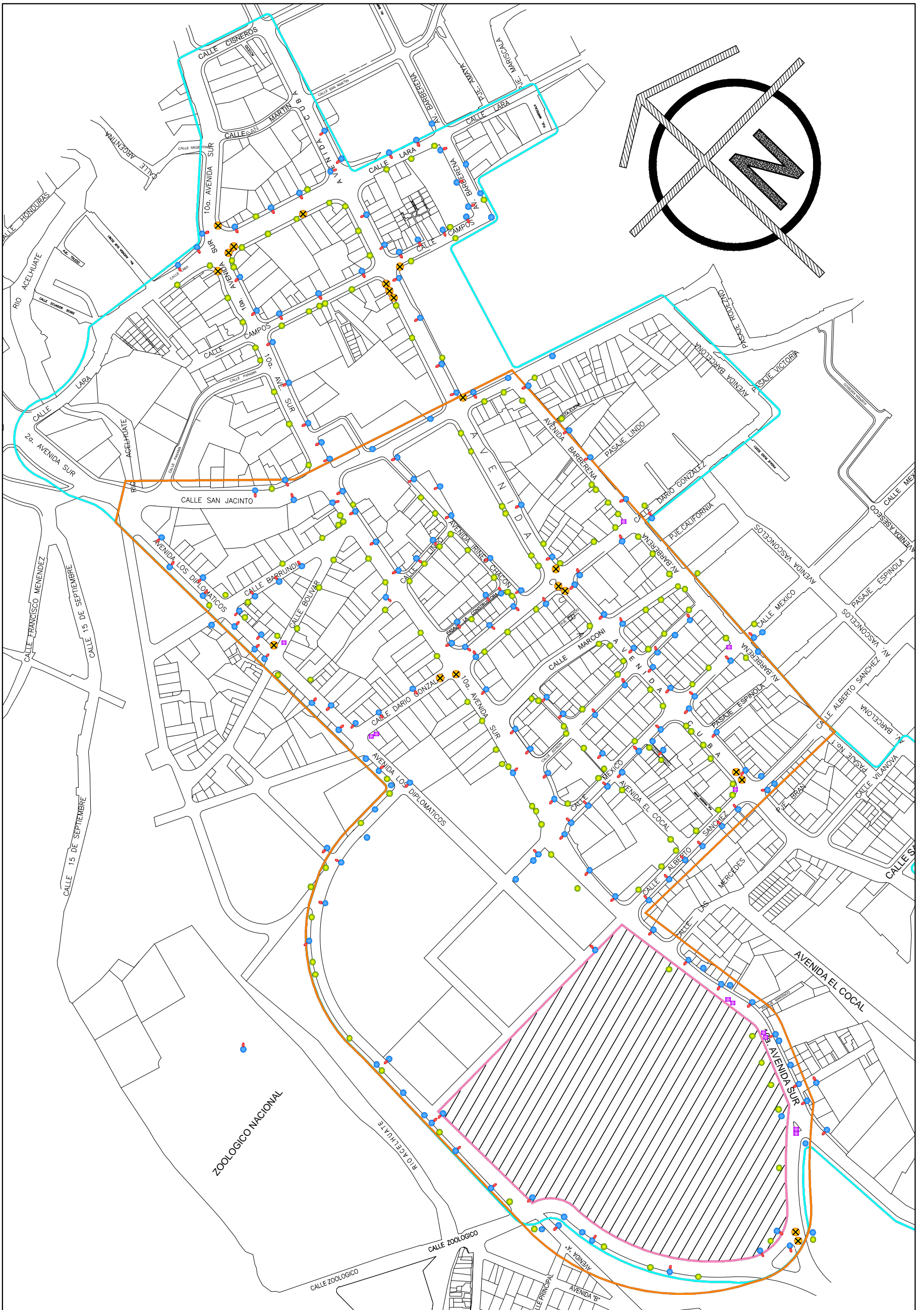
Plano de Infraestructura Eléctrica - Esc.: 1/4000
