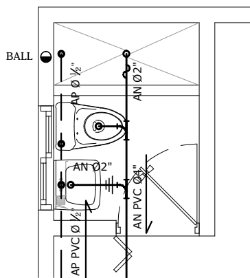
Detalle Baño Dormitorio 1
