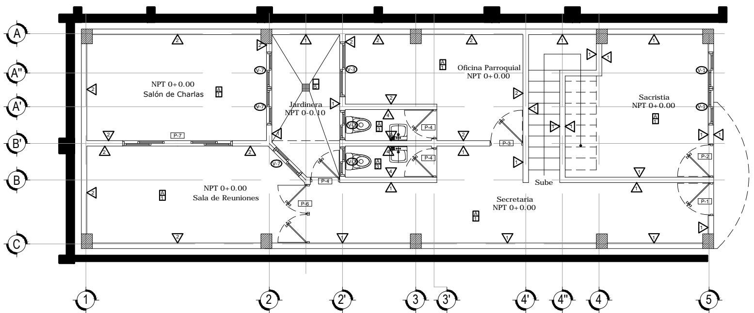
Planta de Acabados - Primer Nivel ESC. 1:100
