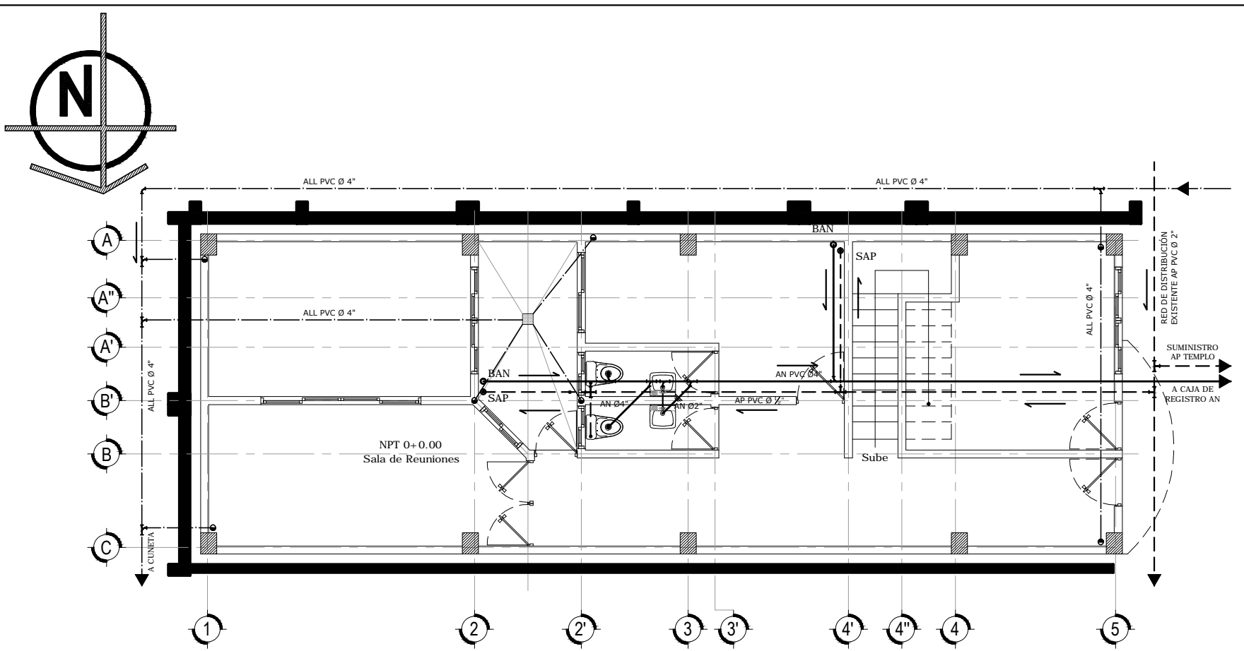
Planta Instalación Hidráulica - Primer Nivel ESC. 1:100
