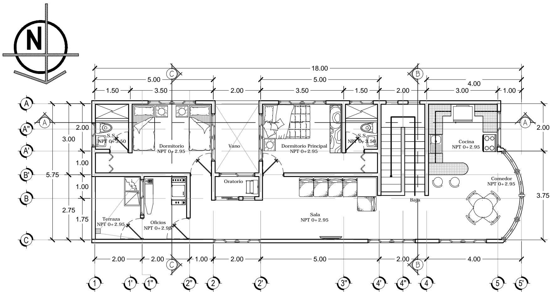
Planta Arquitectónica - Primer Nivel ESC. 1:100
