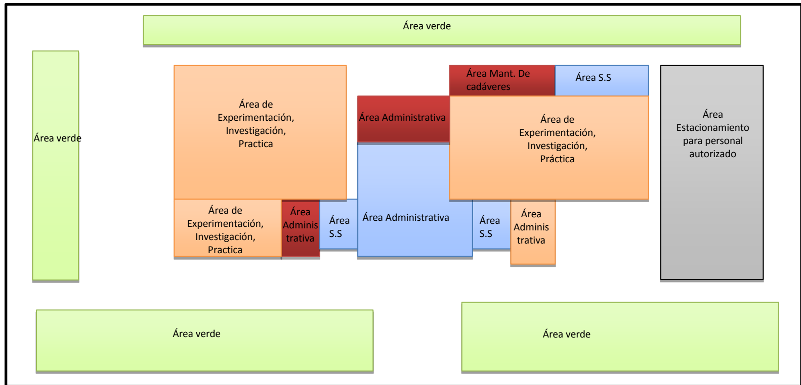
Esquema # 02 Zonificación 1er Nivel.
