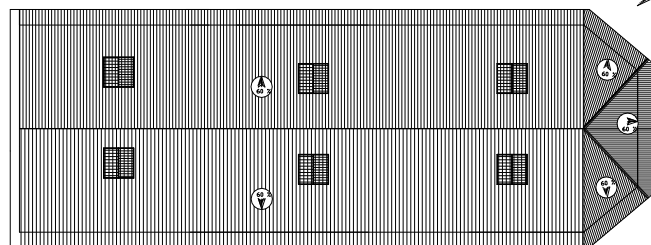
PLANTA DE TECHOS ESC. 1:250
