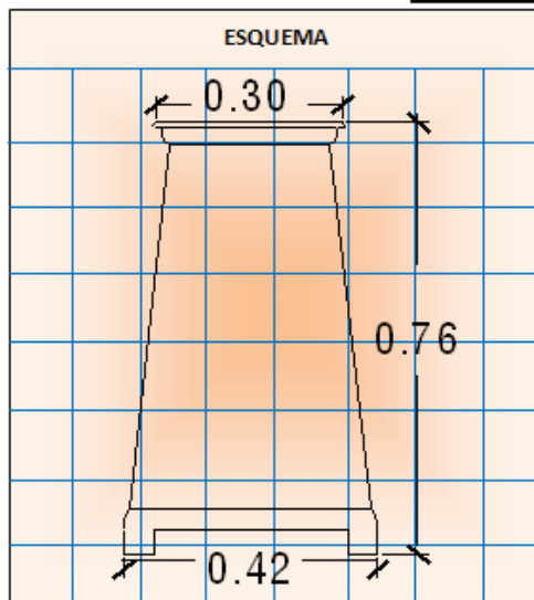
DIMENSIONES
