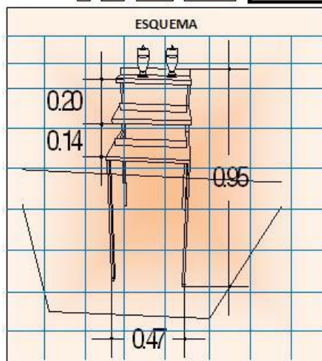
DIMENSIONES
