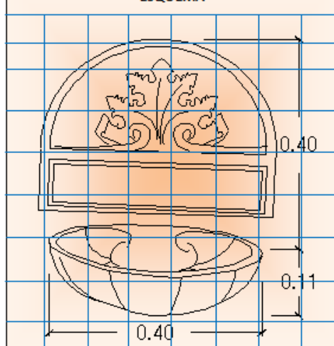
ESQUEMA
