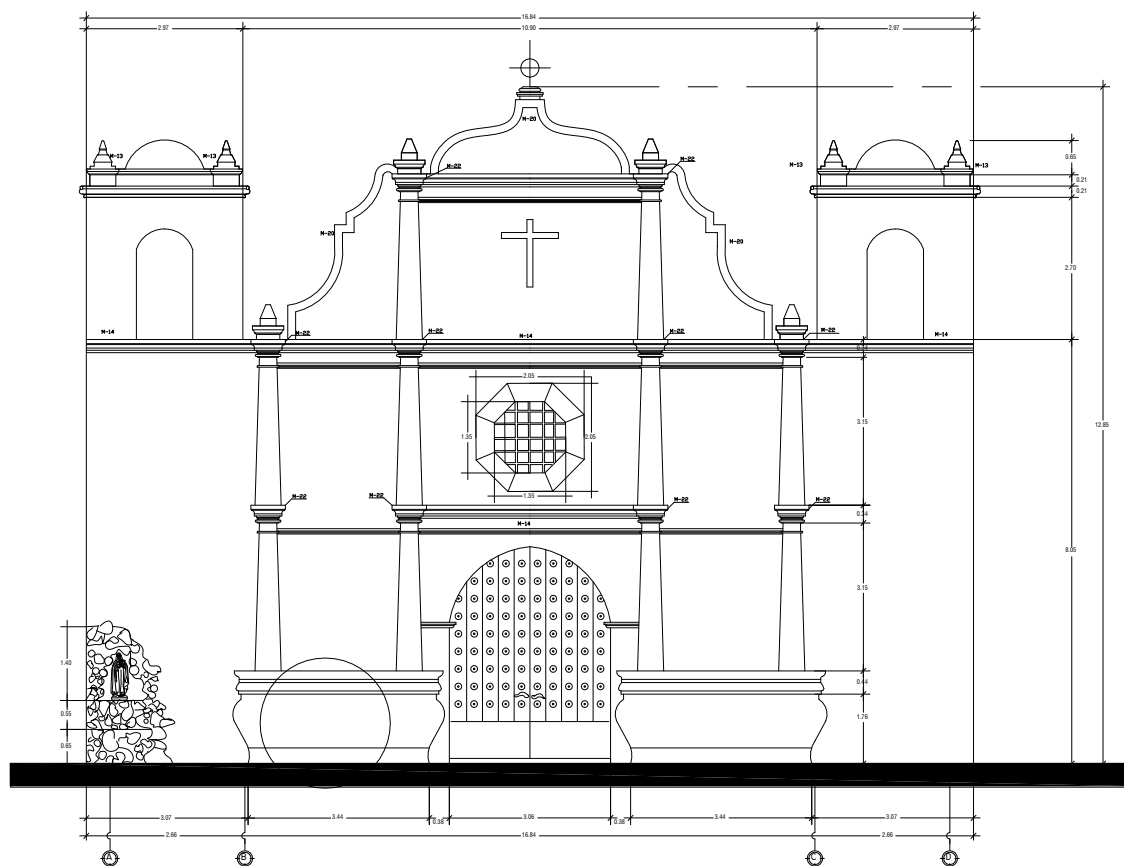
ELEVACION PRINCIPAL ESCALA 1:50
