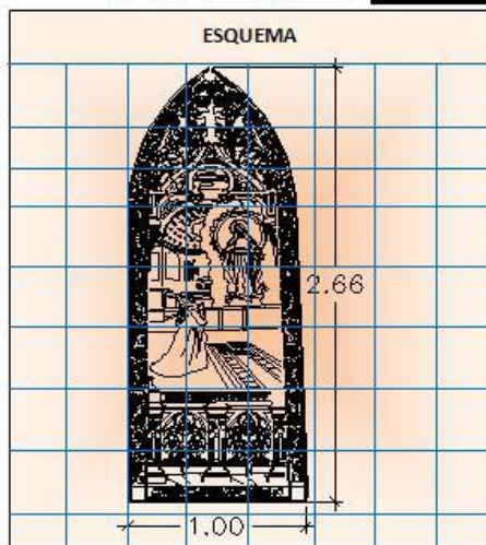
DIMENSIONES
