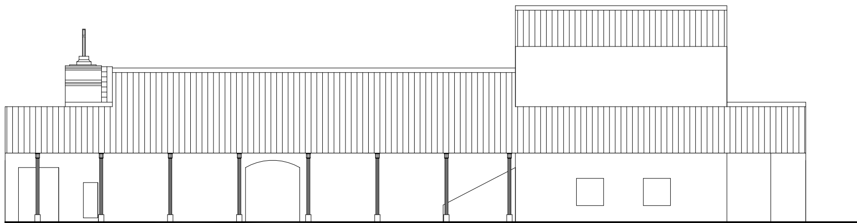
FACHADA SUR
