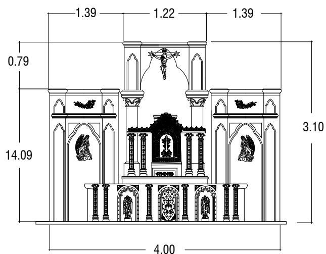
ELEVACION DE RETABLO Esc. 1:100
