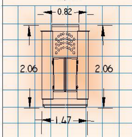
ESQUEMA
