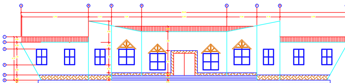
ELEVACION PRINCIPAL EDIFICIO ADMINISTRATIVO
