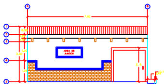
ELEVACION PRINCIPAL AREA DE JUEGOS Esc. 1:100
