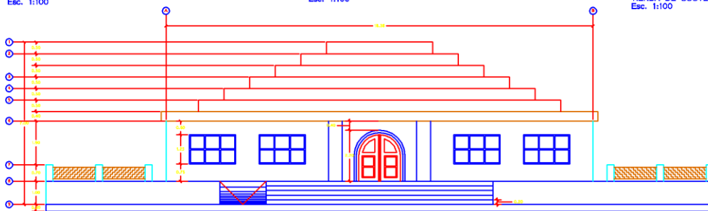
ELEVACION PRINCIPAL RESTAURANTE Esc. 1:100
