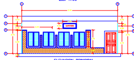
ELEVACION PRINCIPAL CAFETERIA Esc. 1:100
