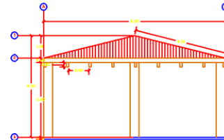
ELEVACION PRINCIPAL BAÑO TÍPICO Esc. 1:100
