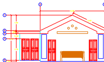
ELEVACION PRINCIPAL BAÑOS Y VESTIDORES
