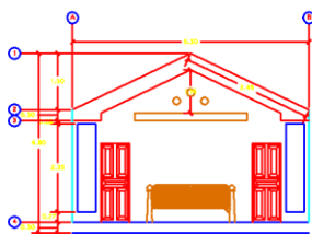
ELEVACION PRINCIPAL BAÑOS
