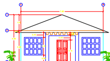
ELEVACION PRINCIPAL BUNGALOWS
