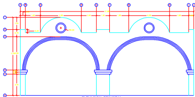
ELEVACION PRINCIPAL ENTRADA PRINCIPAL AL PARQUEO
