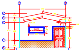
ELEVACION PRINCIPAL CUARTO DE MANTENIMIENTO Esc. 1:100
