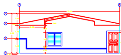
ELEVACION PRINCIPAL DESPACHO DE ACUICULTURA
