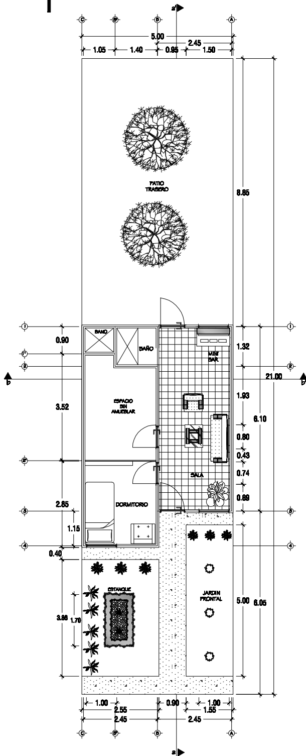
PLANTA ARQUITECTONICA
