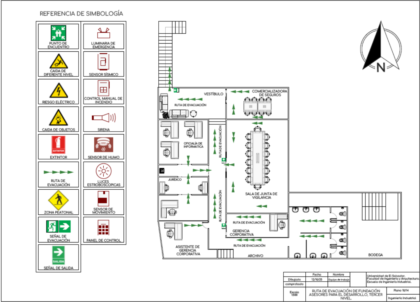
Anexo 11 - Ruta de Evacuación de Fundación Asesores Para El Desarrollo, Tercer Nivel.
