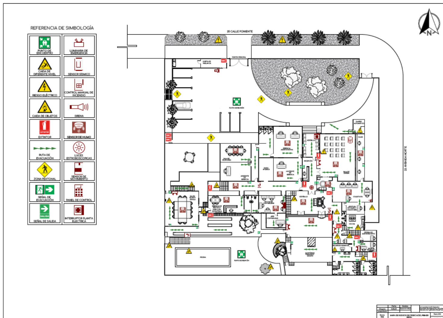
Anexo 4 - Mapa de Riesgos de FEDECASES, Primer Nivel.
