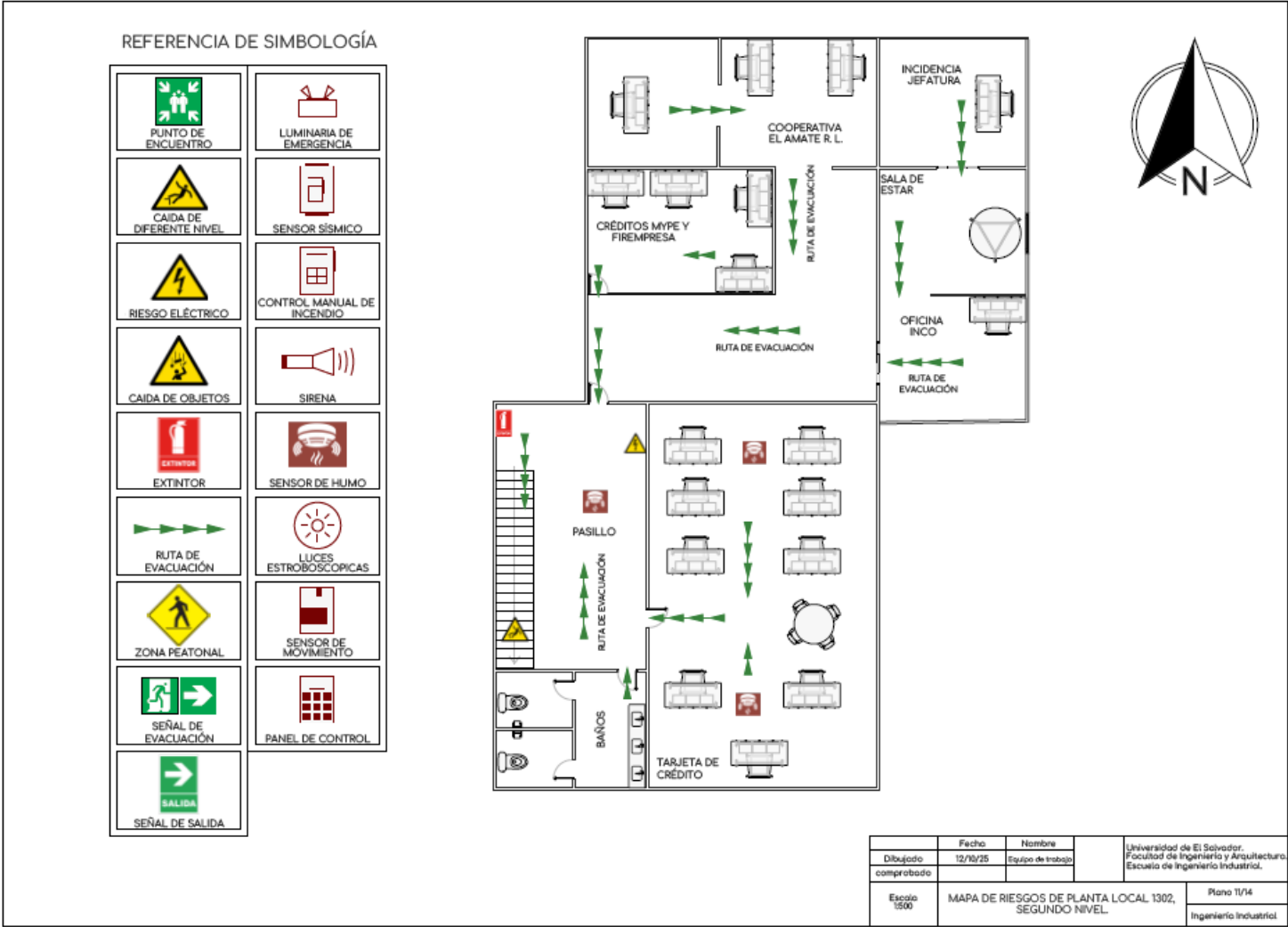
Anexo 14 - Mapa de Riesgos de Planta Local 1302, Segundo Nivel.
