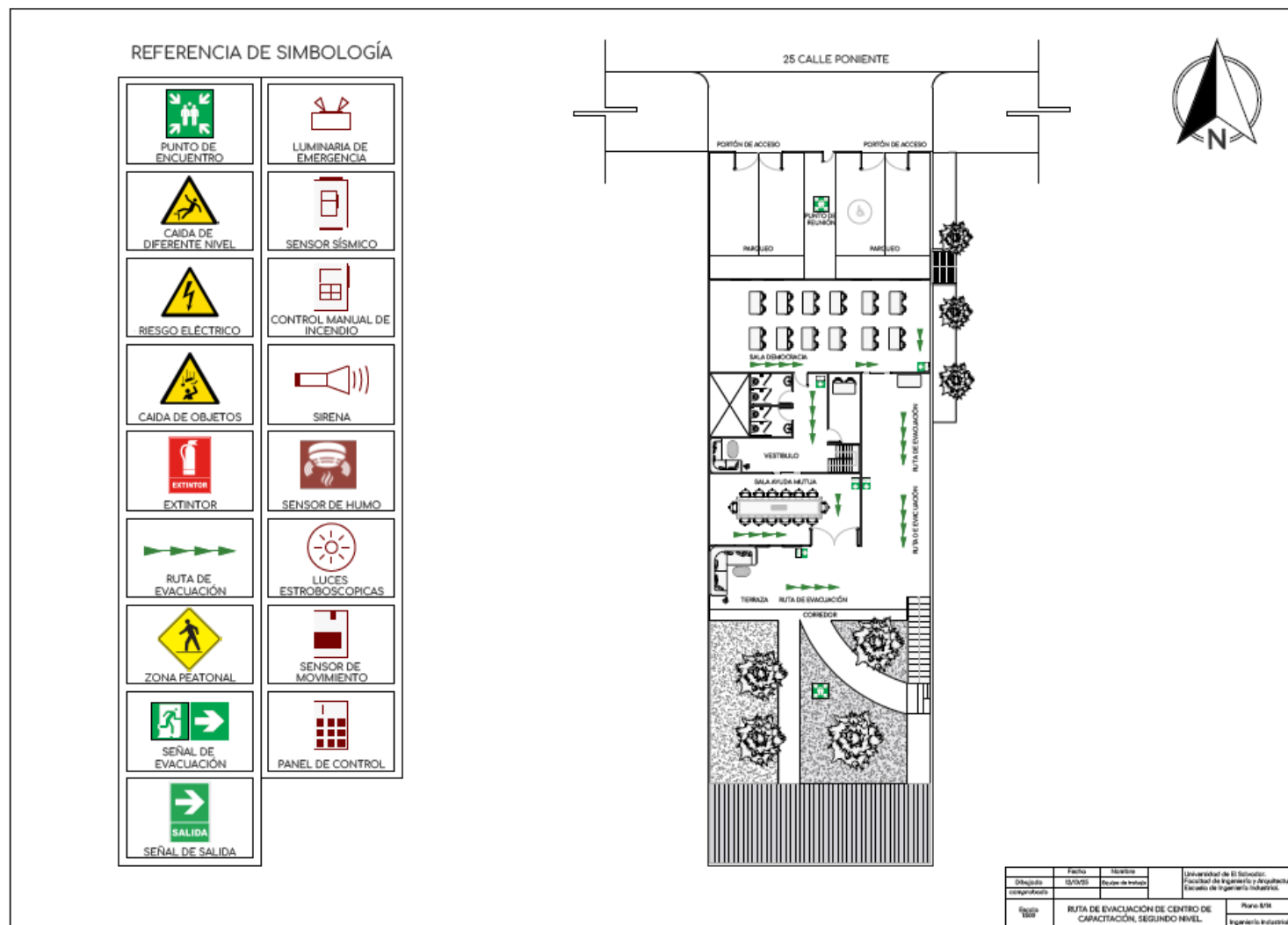
Anexo 9 - Ruta de Evacuación de Centro de Capacitación, Segundo Nivel.
