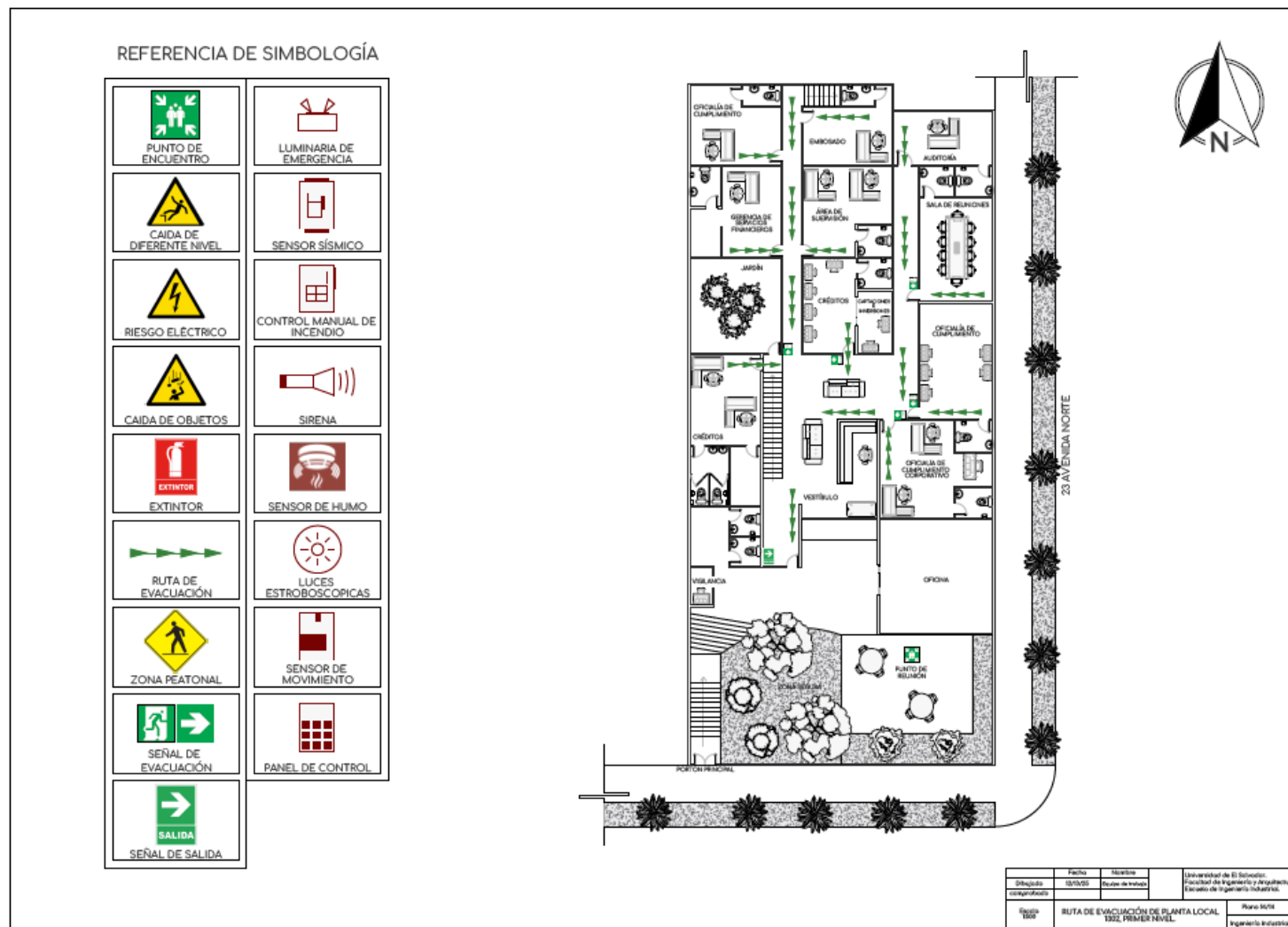
Anexo 13 - Ruta de Evacuación de Planta Local 1302, Primer Nivel.
